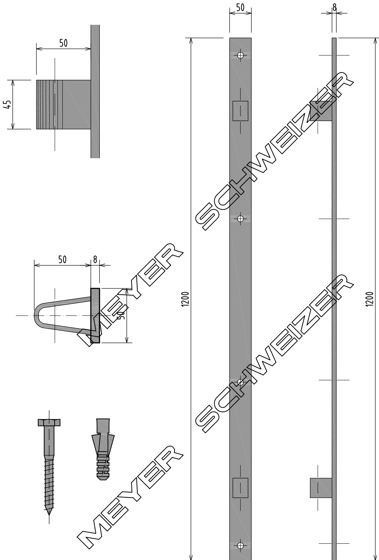
ABSRA-0318 RIEGEL AN WAND DOPPELT
